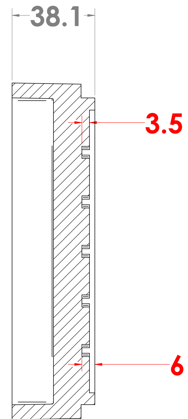
SECTION A-A
