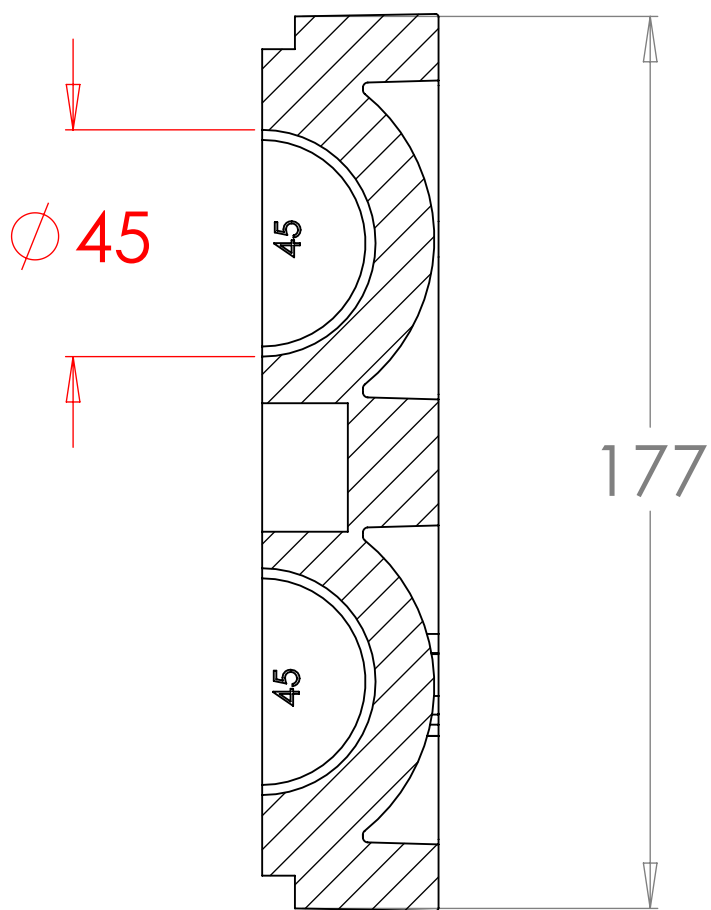
SECTION A-A SCALE 1 : 1.5
