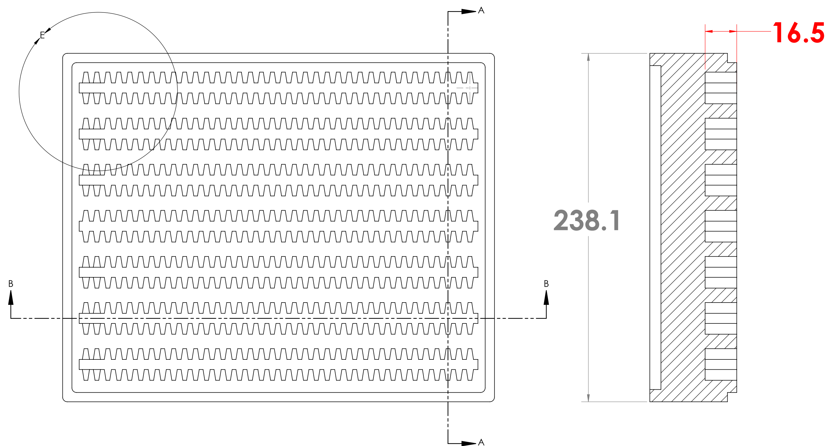
SECTION A-A SCALE 1 : 1.5
