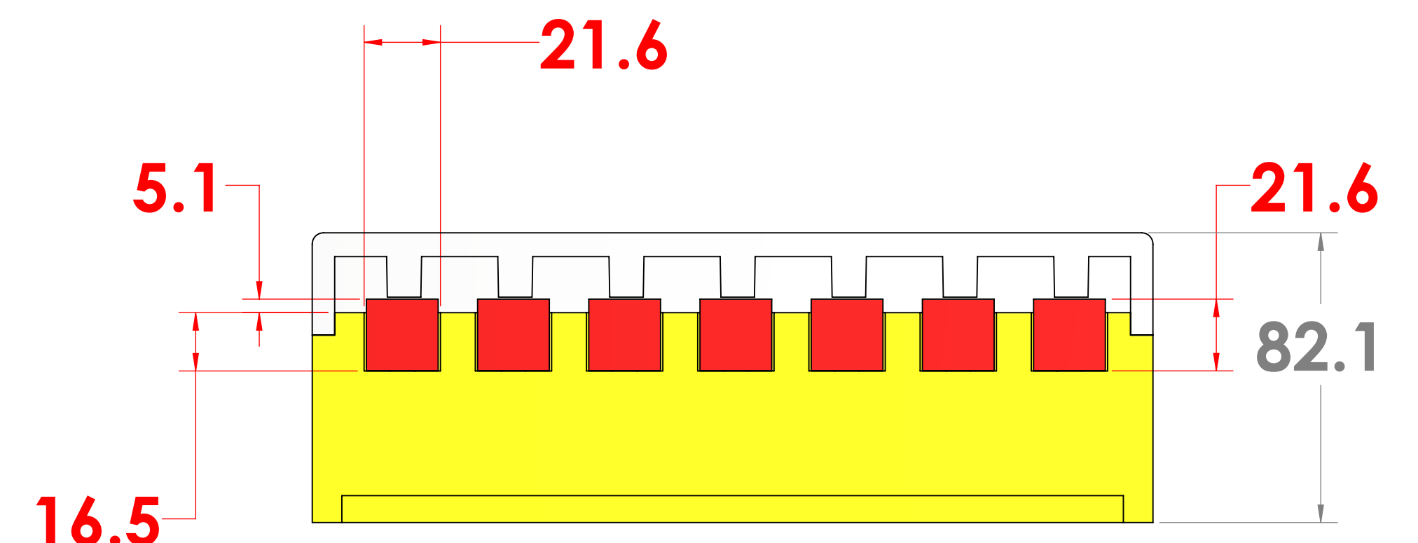
SECTION D-D SCALE 1 : 1.5
