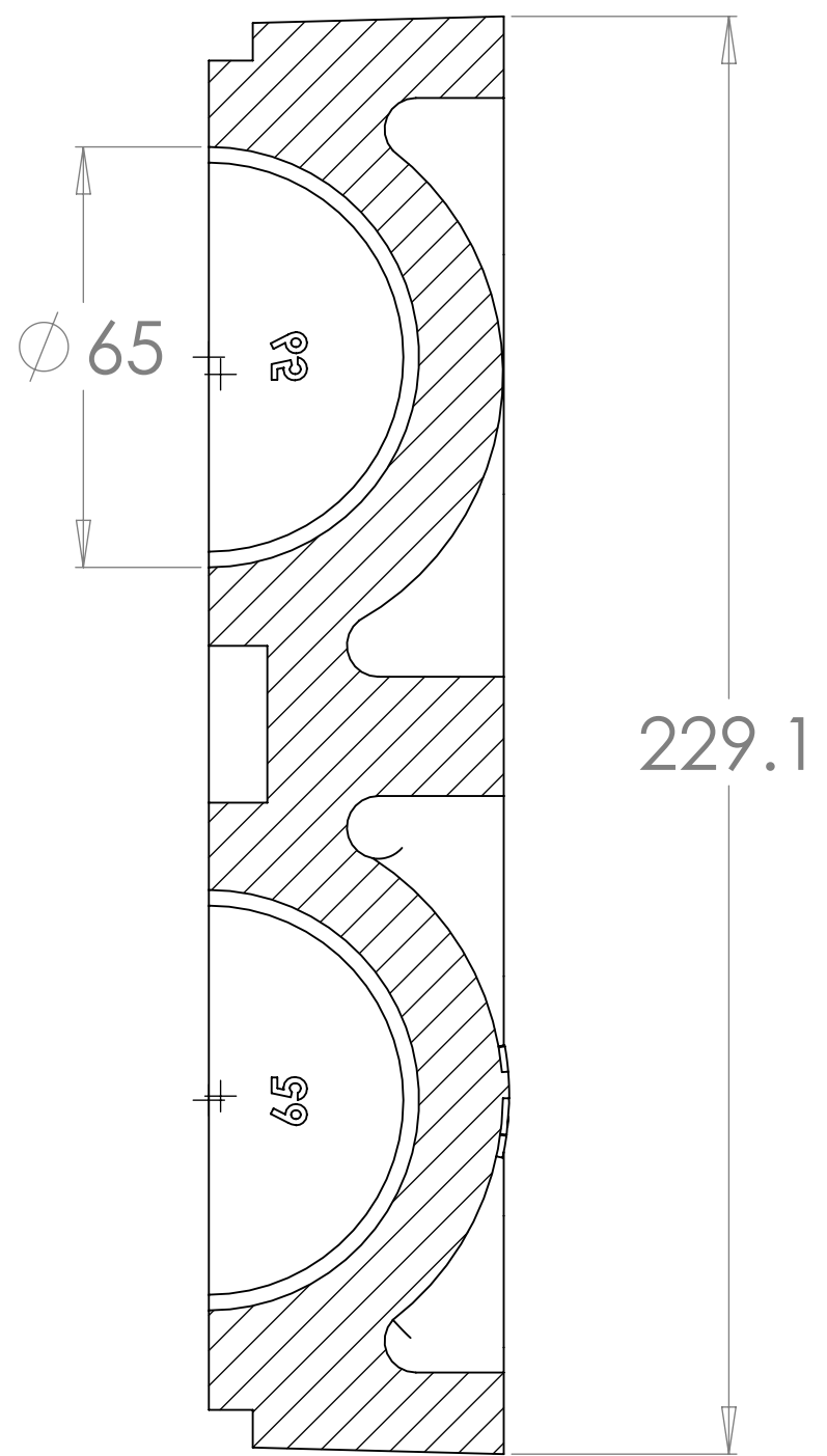
SECTION A-A SCALE 1 : 1.25
