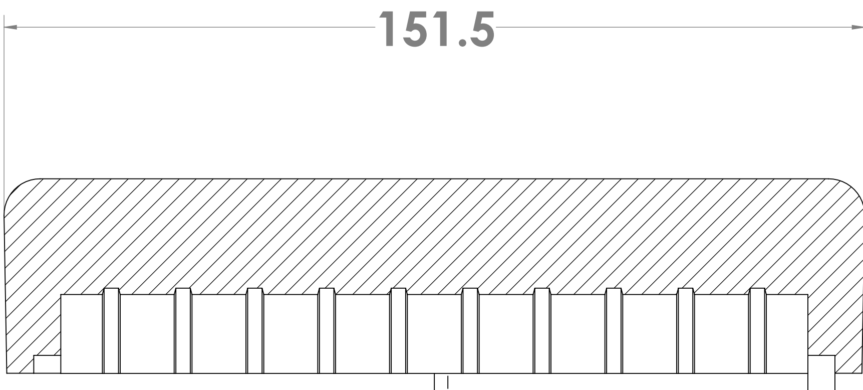
SECTION A-A SCALE 1.5 : 1
