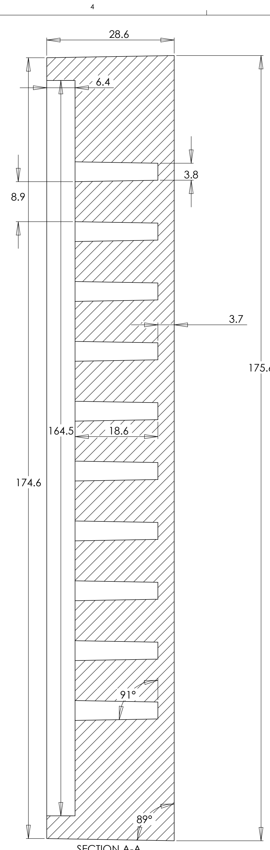
SECTION A-A SCALE 2:1
