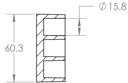
SECTION A-A SCALE 1 : 2
