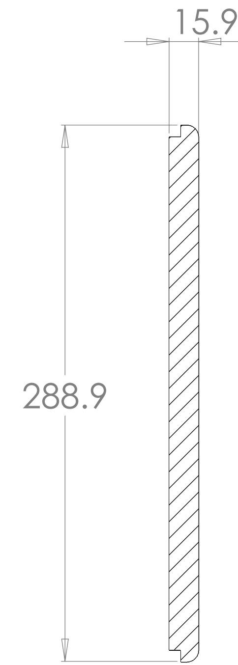
SECTION A-A
