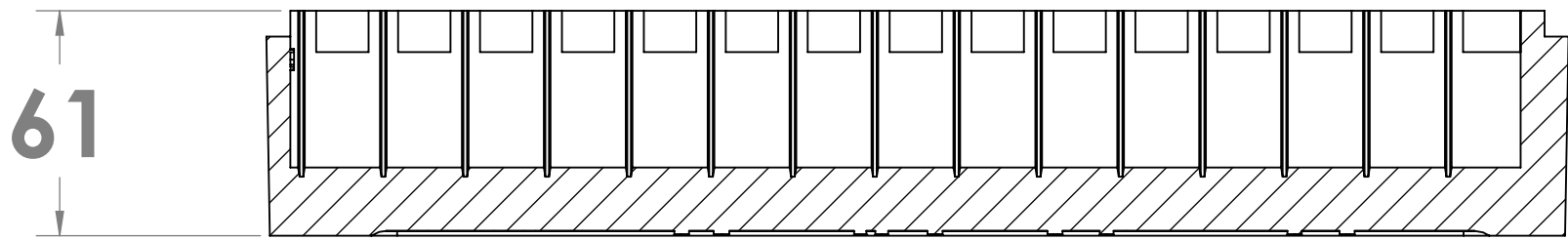
SECTION A-A
