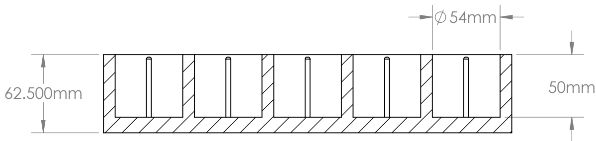
SECTION J-J SCALE 1 : 3
