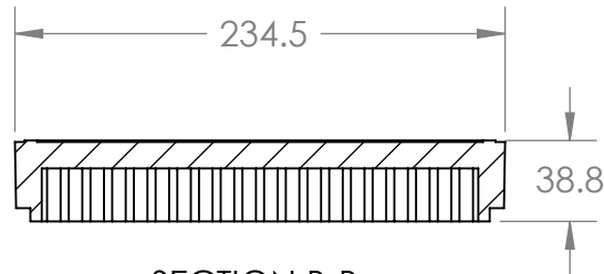
SECTION B-B SCALE 1 : 4
