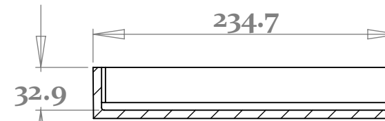
SECTION D-D SCALE 1 : 4
