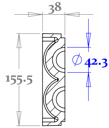
SECTION A-A SCALE 1 : 4
