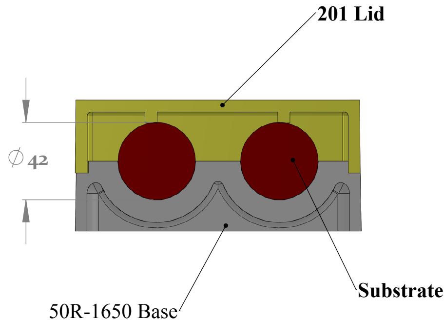
SECTION B-B SCALE 1 : 4
