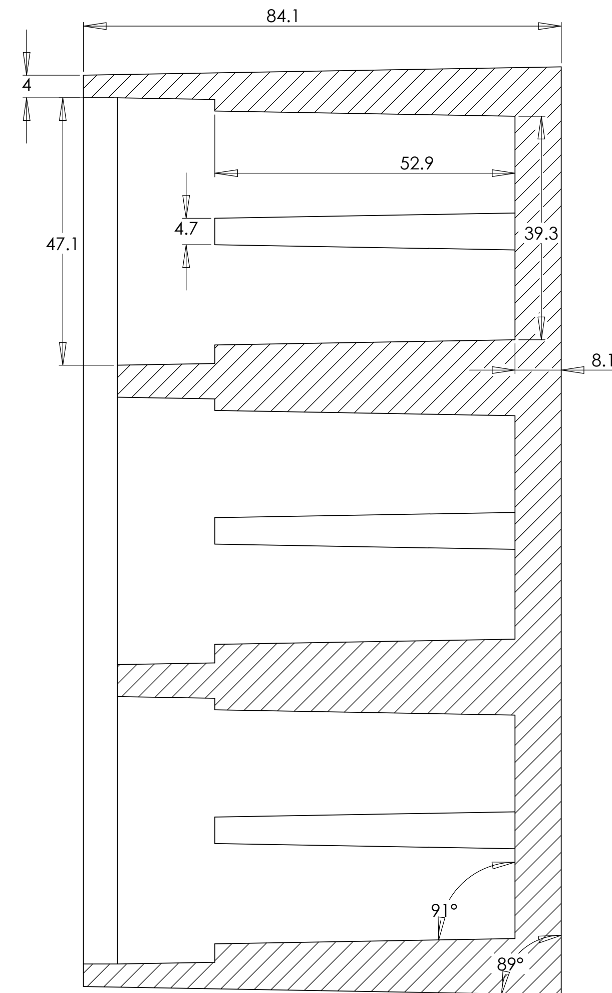
SECTION A-A SCALE 1.5 : 1
