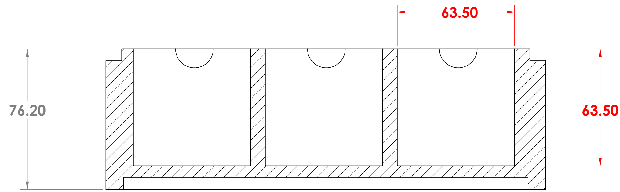
SECTION A-A SCALE 1 : 1.25
