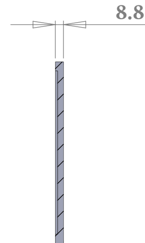
SECTION D-D SCALE 1 : 4
