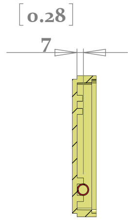
SECTION A-A SCALE 1 : 4
