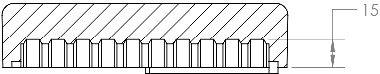
SECTION B-B SCALE 1 : 2
