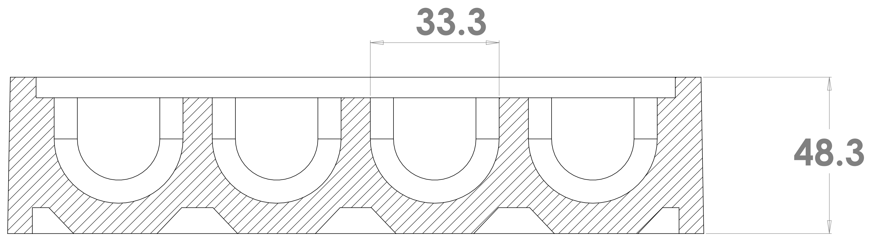
SECTION A-A SCALE 1.5 : 1
